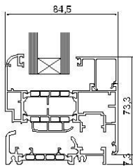
Soglia ribassata anta D1060037
