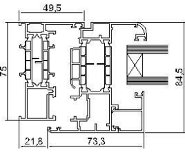
Telaio cassa piana D1060002 + anta D1060037
