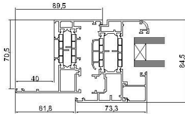
Telaio aletta da 40 mm D1060008 + anta D1060037
