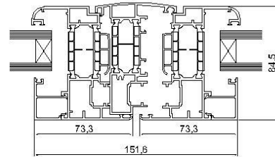
Nodo centrale anta D1060037
