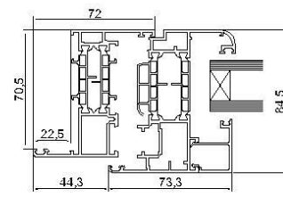
Telaio aletta da 22,5 mm D1060000 + anta D1060037
