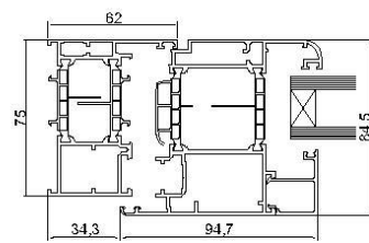
Telaio cassa piana D1060021 + anta portoncino D1060038
